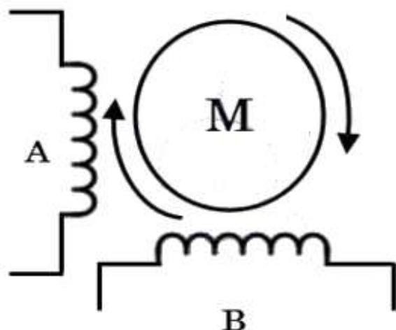
Motore passo-passo bipolare a 2 fasi
