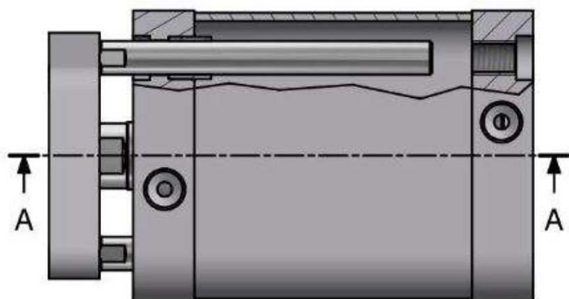
Esempio di cilindro compatto con anti rotazione
